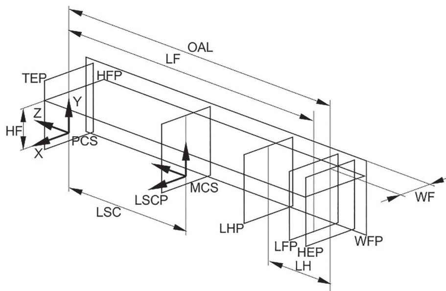
Figure 5 — Exemple de plans de références pour la conception
