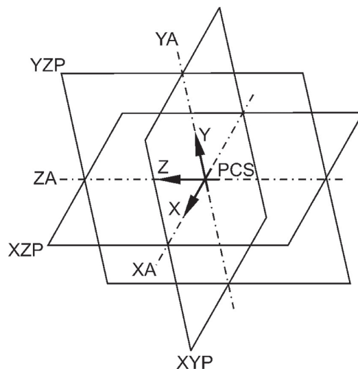
Figure 1 — Système de coordonnées principal
